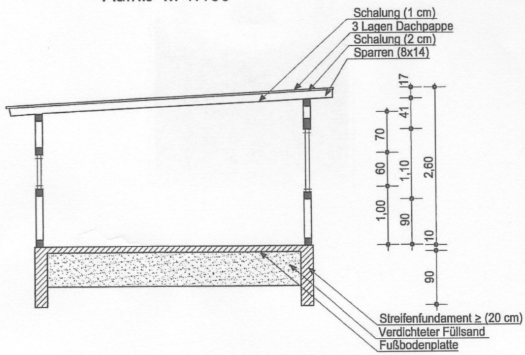
Aufriß M 1:100
