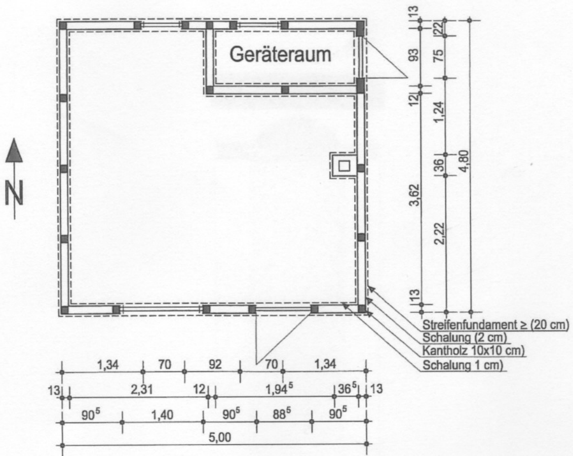
Grundriß M 1:100
