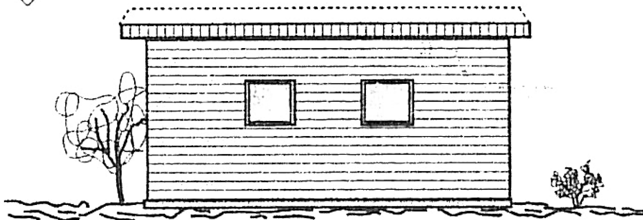
Nord-Ansicht M 1:100
