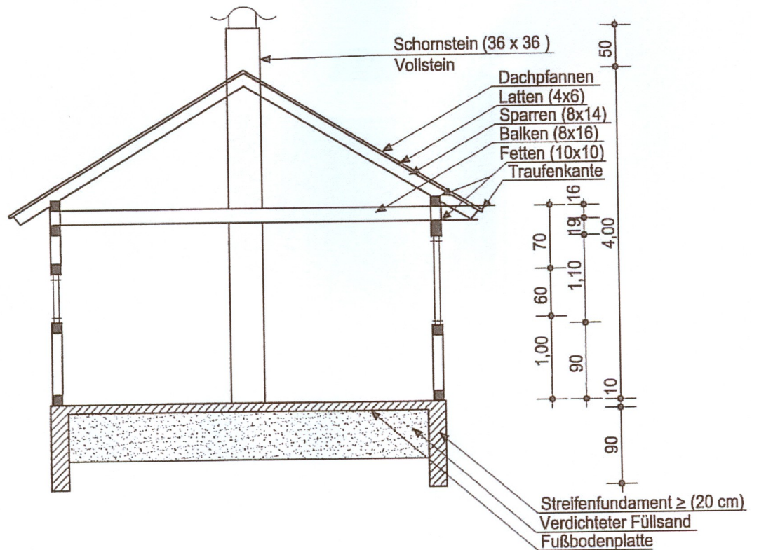
Aufriß M 1:100
